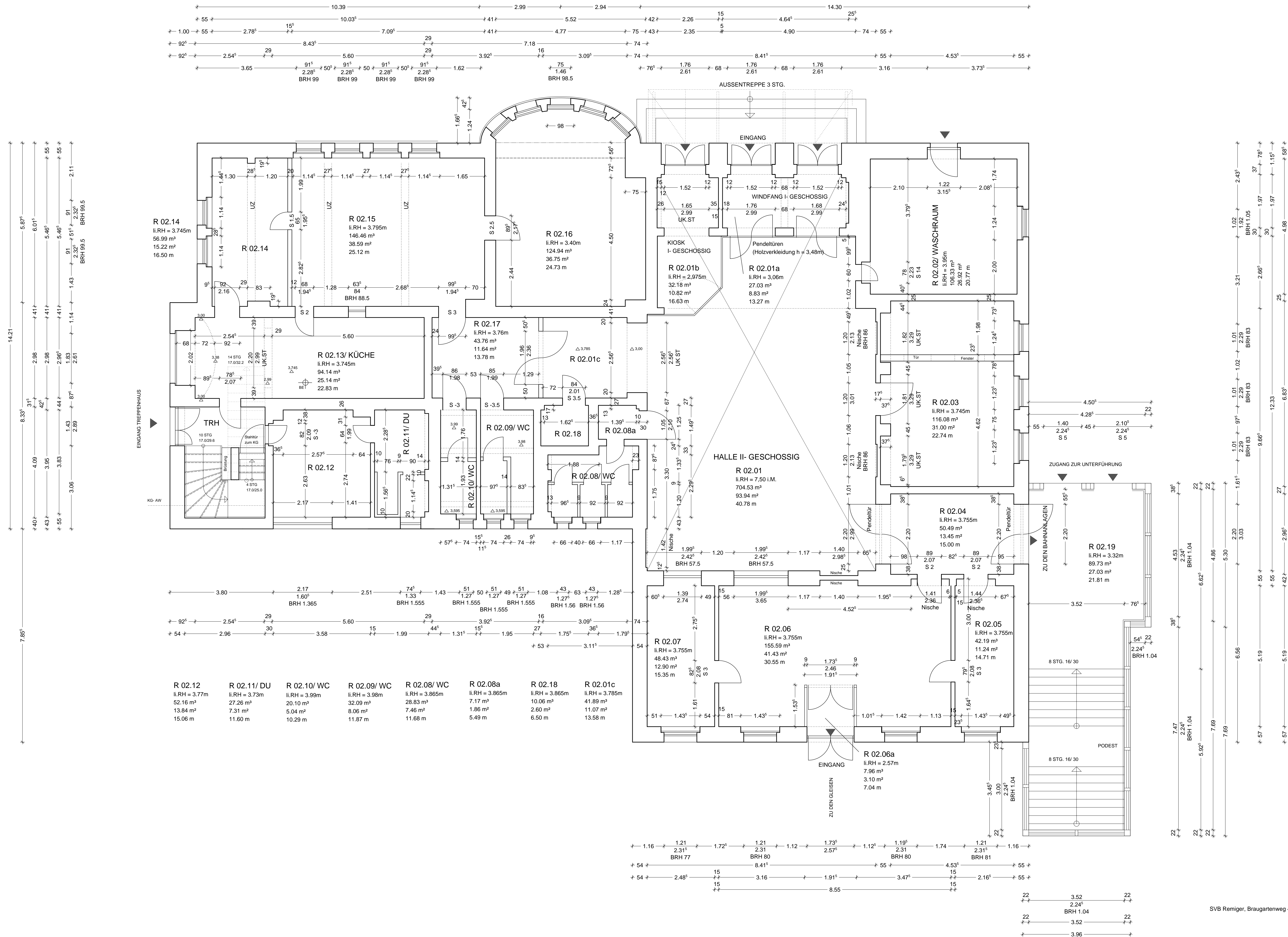
Bestandsplanung Grundriss ERDGESCHOSS 1 : 50
